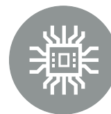
AI Acceleration
